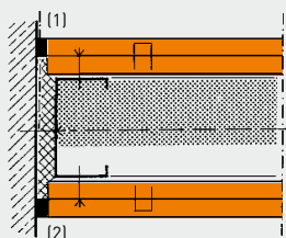
Wand- en plafondaansluitingen met dubbele fermacell beplating
